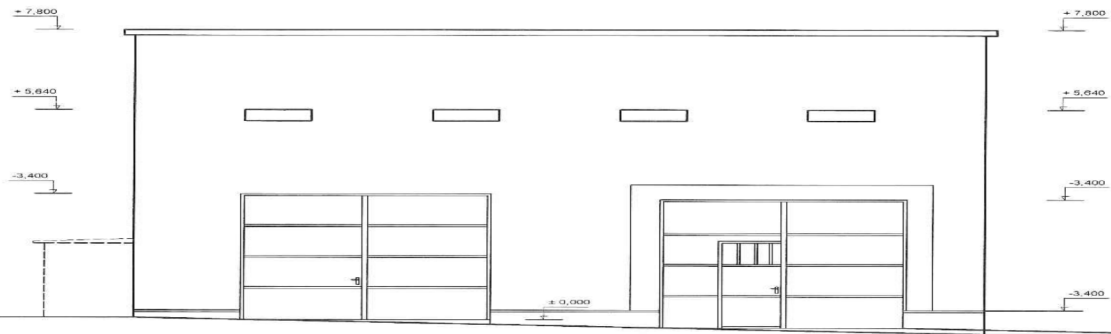
POHLAD JUŽNÝ
